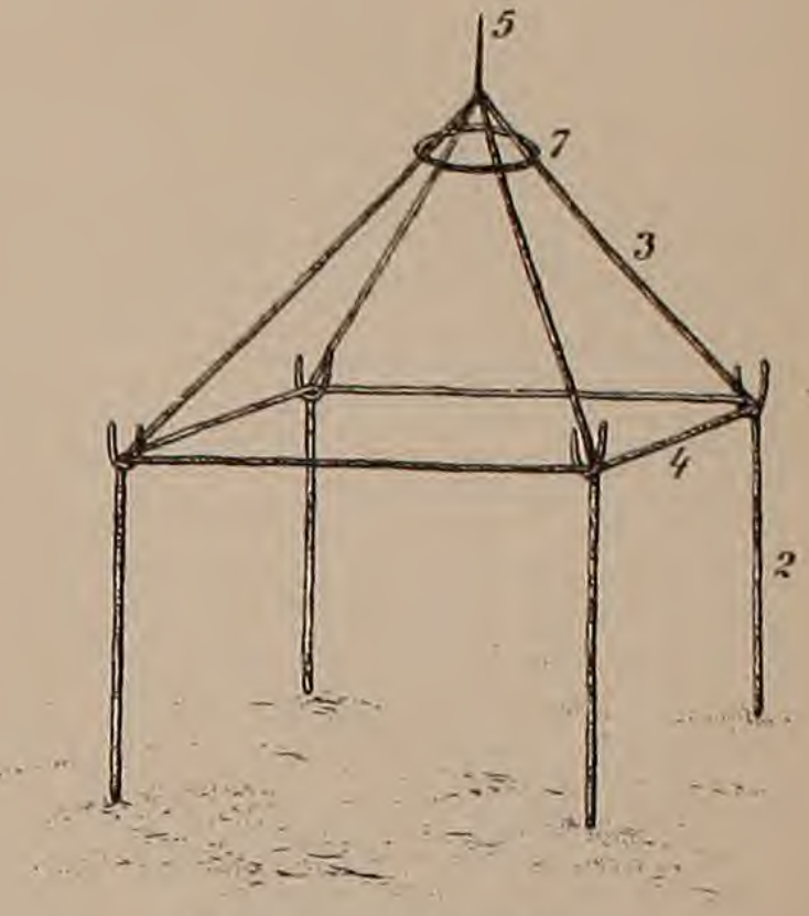
Akposso. Dachgerippe
